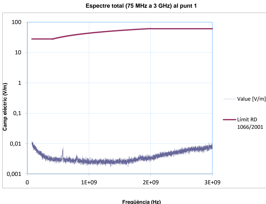
Figura 1. Valors de camp elèctric obtinguts per les freqüències entre 75 MHz i 3 GHz al punt 1.
