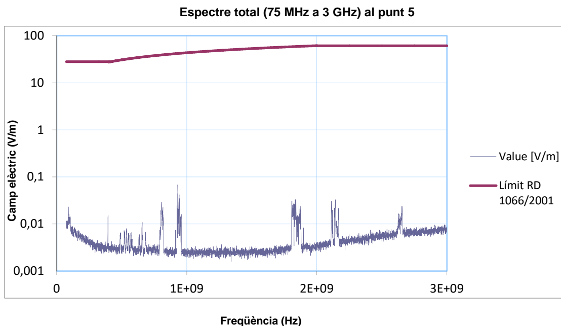
Figura 5. Valors de camp elèctric obtinguts per les freqüències entre 75 MHz i 3 GHz al punt 5.
