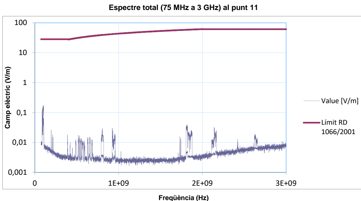
Figura 11. Valors de camp elèctric obtinguts per les freqüències entre 75 MHz i 3 GHz al punt 11.
