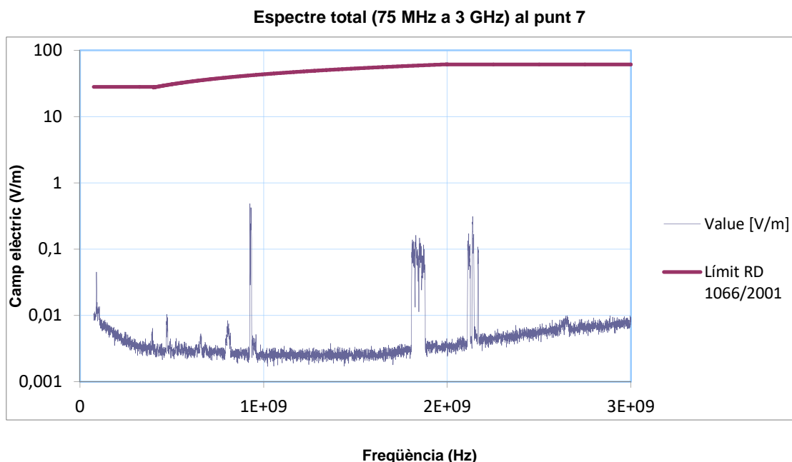
Figura 7. Valors de camp elèctric obtinguts per les freqüències entre 75 MHz i 3 GHz al punt 7.
