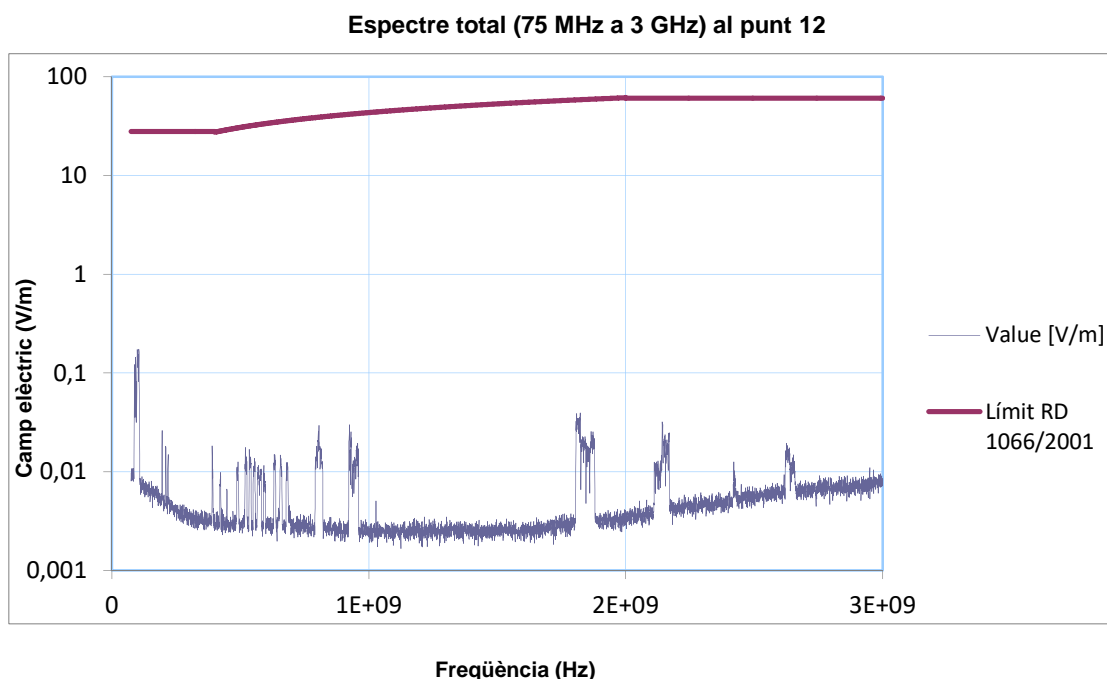
Figura 12. Valors de camp elèctric obtinguts per les freqüències entre 75 MHz i 3 GHz al punt 12.
