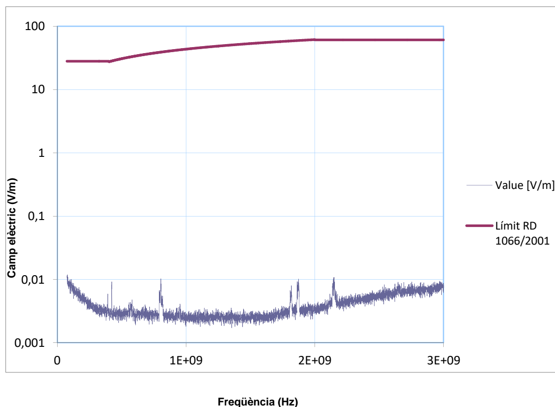
Figura 2. Valors de camp elèctric obtinguts per les freqüències entre 75 MHz i 3 GHz al punt 2.
