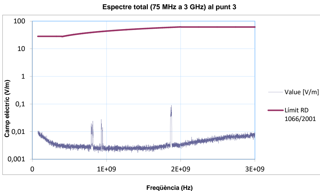
Figura 3. Valors de camp elèctric obtinguts per les freqüències entre 75 MHz i 3 GHz al punt 3.
