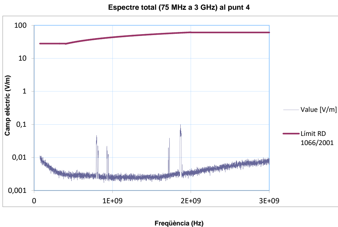
Figura 4. Valors de camp elèctric obtinguts per les freqüències entre 75 MHz i 3 GHz al punt 4.
